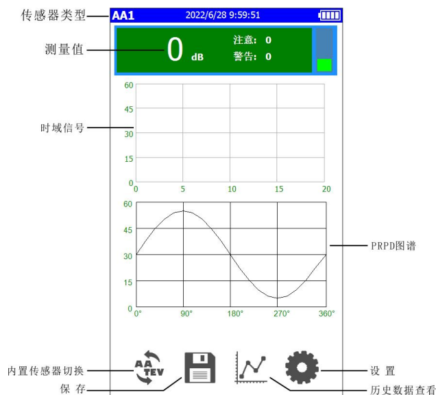
测试界面
