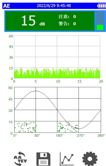
时域信号波形和 PRPD 相位图谱
