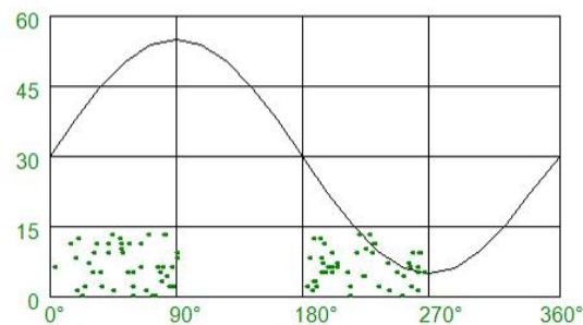
PRPD 图谱
