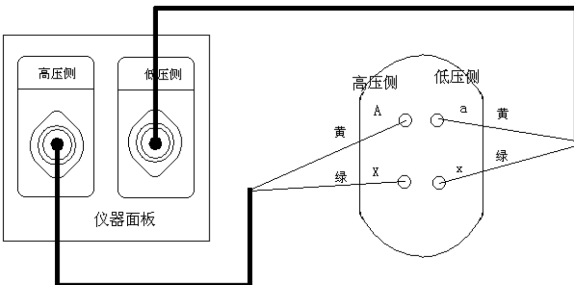
图十五、单相变压器的测试接线
